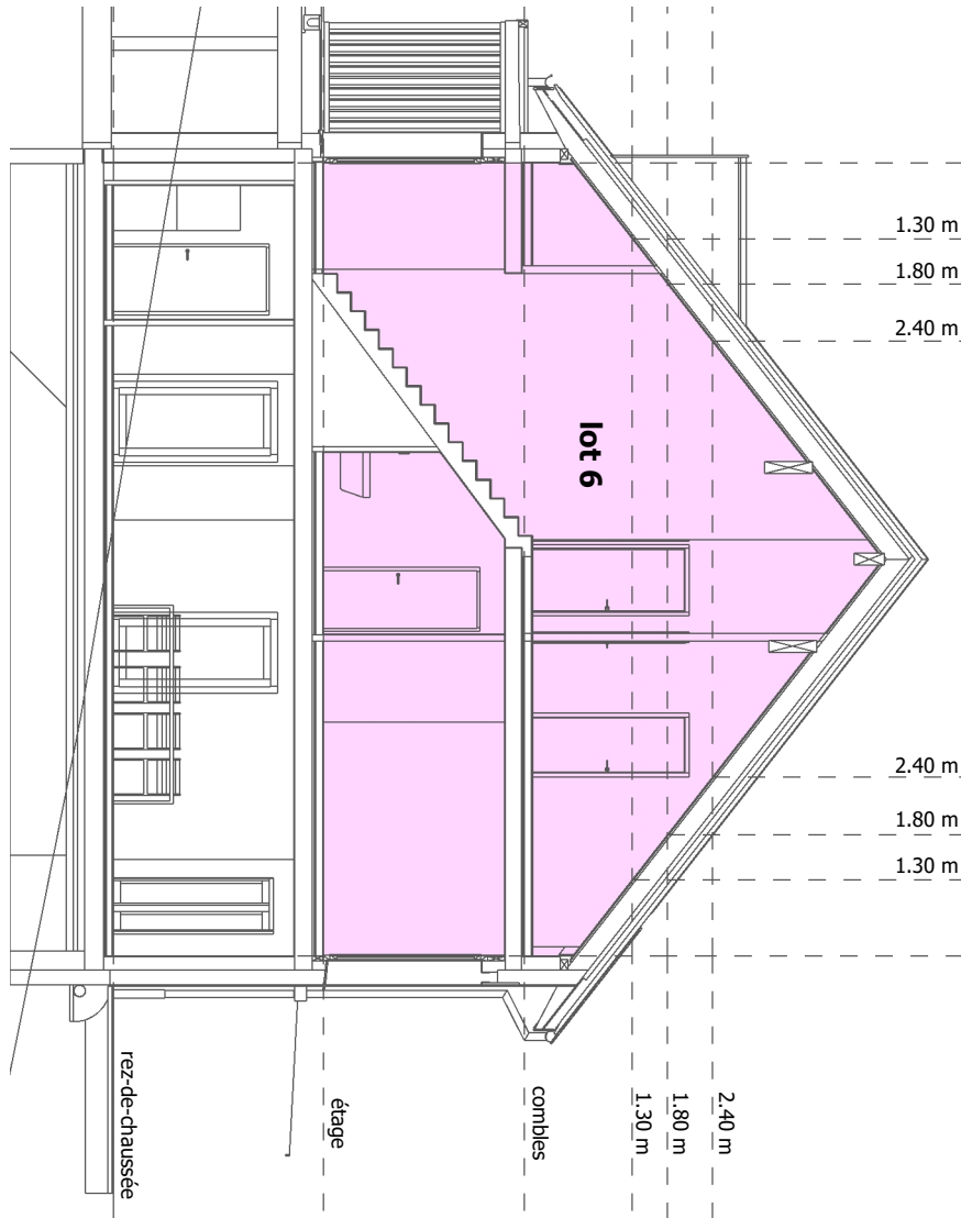
Coupe B-B'
