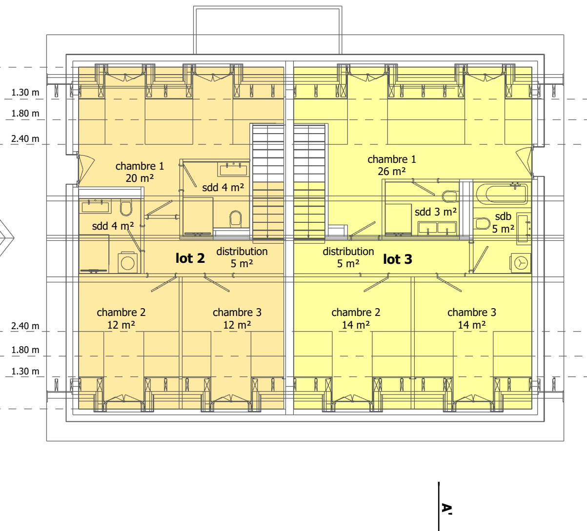
Plan des combles
